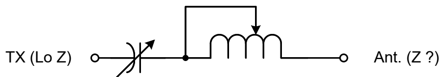
Antenna Tuner - "Series" Type Bloc d'Accord d'Antenne – "Série" ( ARRL Handbook )
